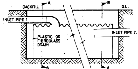
LONGITUDINAL SECTION
