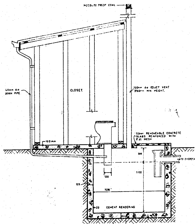
SECTION A-A.
