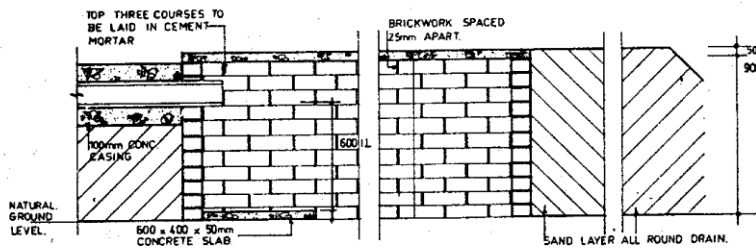
LONGITUDINAL SECTION.
