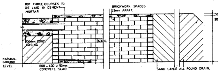
LONGITUDINAL SECTION.
