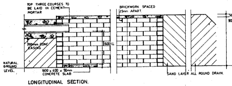
LONGITUDINAL SECTION.
