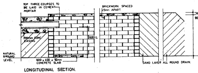
LONGITUDINAL SECTION.
