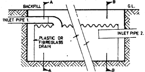
LONGITUDINAL SECTION
