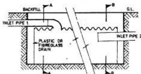
LONGITUDINAL SECTION
