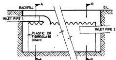
LONGITUDINAL SECTION
